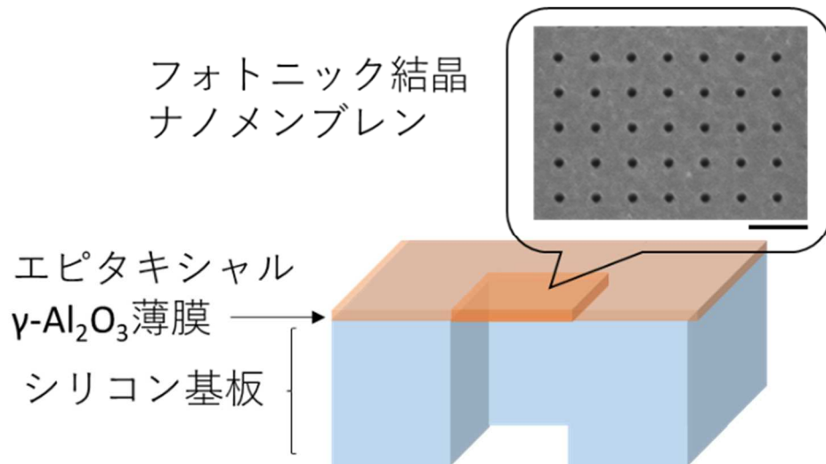
図 2: 作製したフォトニック結晶ナノメンブレンの模式図と電子線顕微鏡像。スケールバーの長さは1 \mu\text{m} 。
