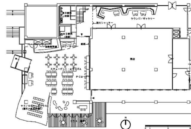
1F 平面図 1/500
